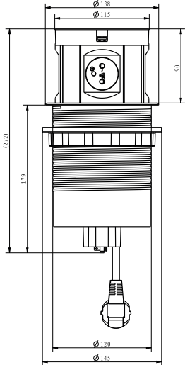
VUE DE FACE – OUVERT
