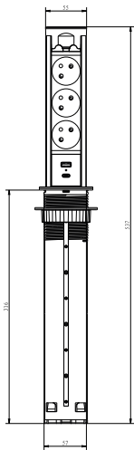
VUE DE FACE - OUVERT
