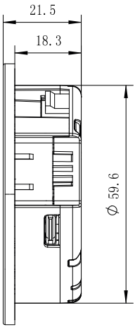
VUE LATÉRALE
