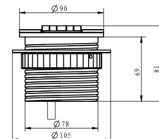
VUE LATÉRALE
